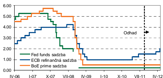
Graf: Kľúčové úrokové sadzby Graf: 3M Euribor, Libor USD and Libor GBP
